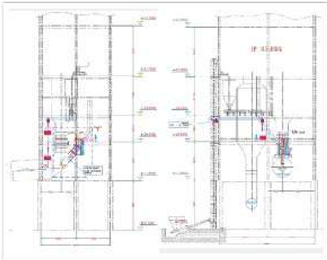
Gambar 2. Desain Chute Fasilitas Pemanfaatan Ban Bekas di Kiln
