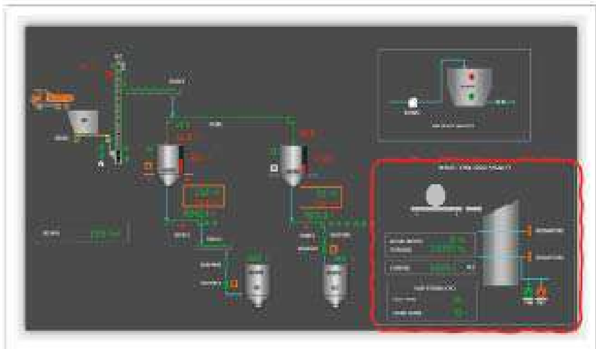
Gambar 5. Tampilan Fasilitas Pemanfaatan Ban Bekas di Monitor CCR Operator Setelah Inovasi
